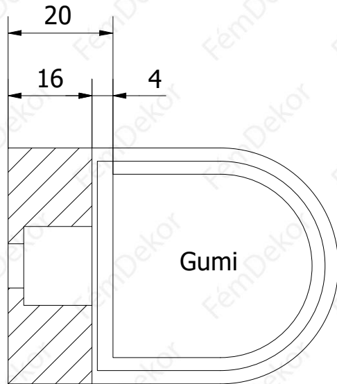
A-A (1:1)
