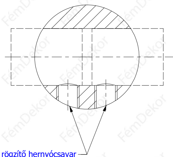
A-A ( 2 : 1 )
