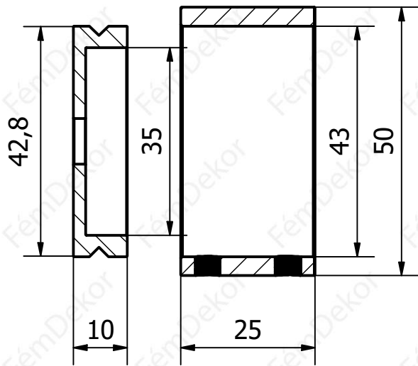
A-A (1 : 1)
